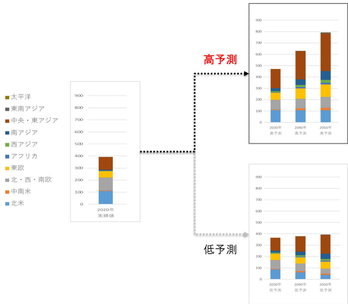
【原子力発電の将来予測（実績および予測 百万kW）】
